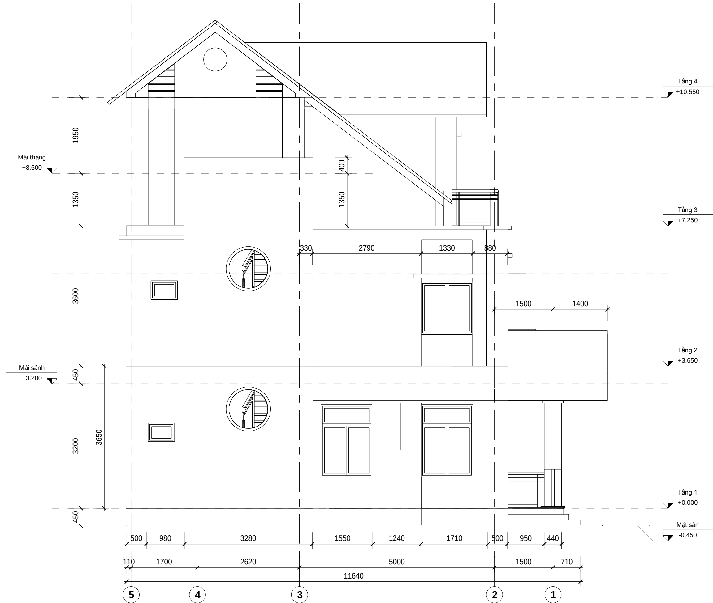
MẶT ĐỨNG TRỤC 5-1
