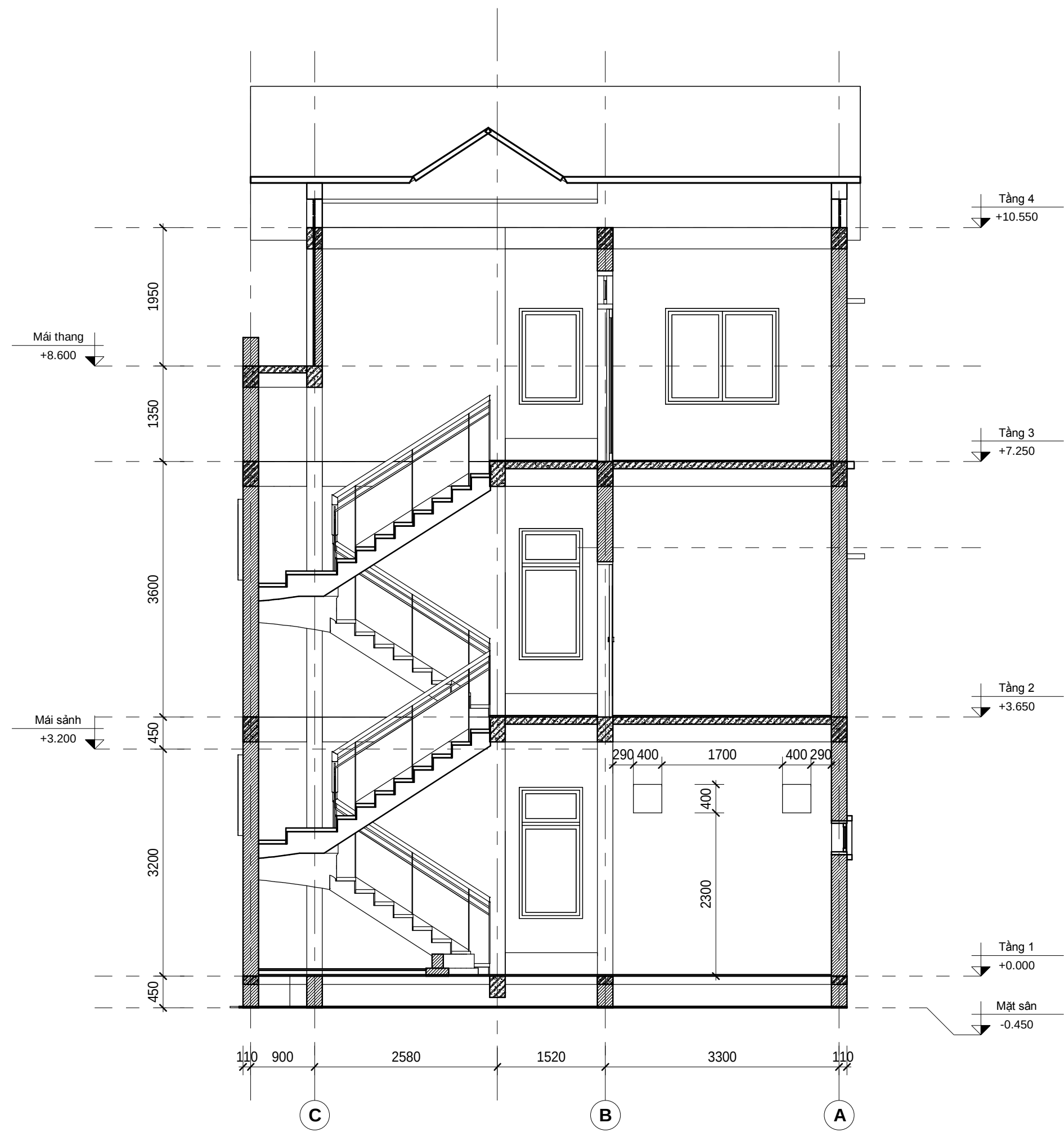
MẶT CẮT A-A
